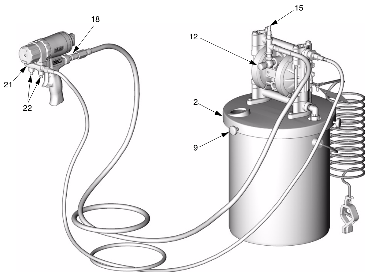
FIG. 3. 248229 Pail Kit
